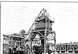
Мобильный асфальтобетонный завод фирмы Lintec CSD-2500 (пр-во Германия)
